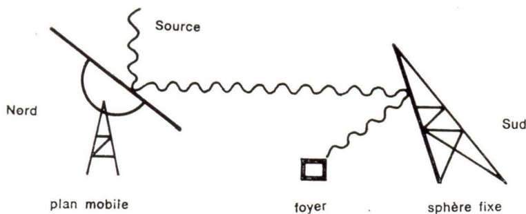
Coupe verticale du grand radiotélescope de Nançay.
