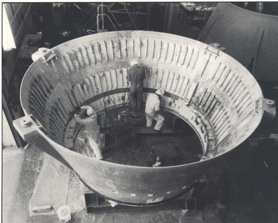
Opbygning af »skørtet« til rumfærgen.
