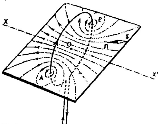
- Le champ magnétique d'un courant circulaire
