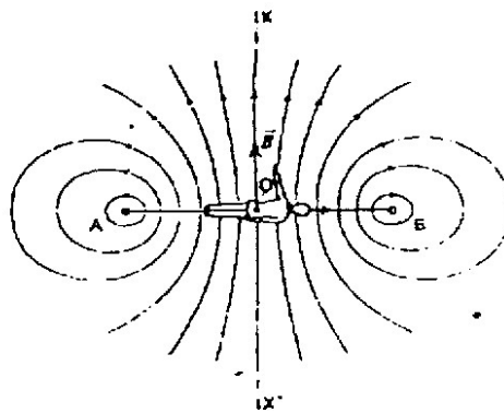
- Les lignes d'induction d'un courant circulaire
