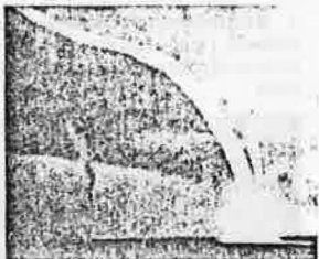
Parfois, c'est à proximité de la surface des eaux que se forment d'inhabituels phénomènes atmosphériques (ici une trombe) susceptibles de faire naître chez quelques témoins une vision insolite (Cliché Météorologie nationale).
