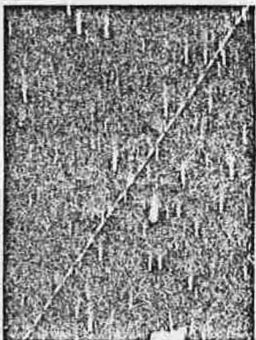
Autre exemple fréquent de méprise, là encore facilement identifiable par les experts : les objets satellisés autour de la Terre. Cette ligne oblique pointillée est, en fait, la trace de passage de l'étage supérieur d'une fusée porteuse de satellite artificiel, étage qui pivote sur lui-même assez rapidement (ici deux fois par seconde) ce qui s'accompagne de variations d'éclat. La trace parallèle, sur la gauche, moins bien visible, est celle du satellite placé sur orbite par cette fusée.
