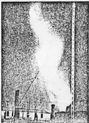
Les aurores polaires sont généralement étudiées dans la région des pôles de la Terre mais en période d'agitation magnétique extrême, elles ont pu être visibles jusqu'à Paris.
