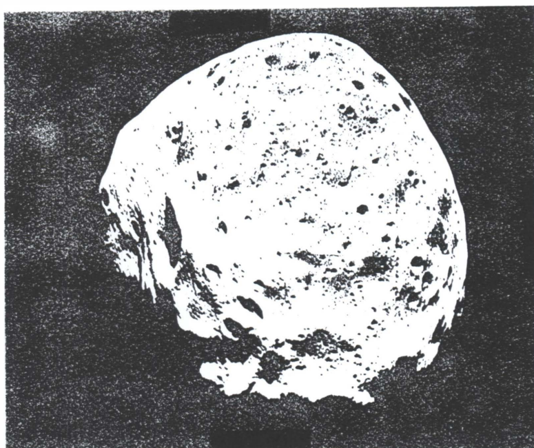
"Phobos" (NASA)
