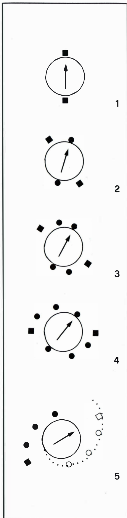
La sequenza mostra il generarsi di una galassia con la successiva elezione delle masse. In base al meccanismo esposto dalla teoria, il generarsi di segmenti di spirale è un fatto conseguente la rotazione del sistema di riferimento.
