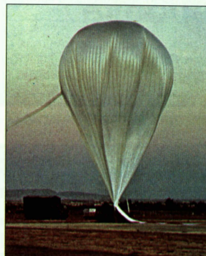
Un pallone sonda in fase di gonfiaggio.
