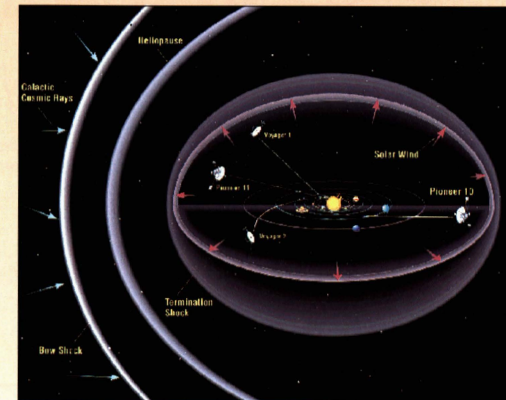
Le traiettorie delle sonde Voyager e Pioneer fuori del Sistema Solare.
