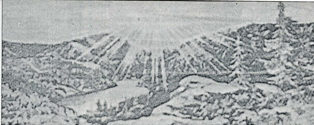
Dette er en tegning av såkalt halogen-fenomen. Vi ser et halofenomen ved lav solhøyde - med lysende ring og bisoler i vinkelavstand av 22 grader fra sola.
