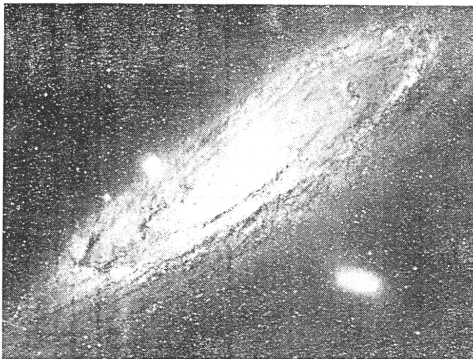
Denne store spirallåke finner vi i stjernebildet Andromeda og den ligner mye på vår Melkevei. Diameteren på denne galaksen (= stjernesystem) er 52.200 lysår. Den store lysende flekken på bildet er en drabant-galakse.
