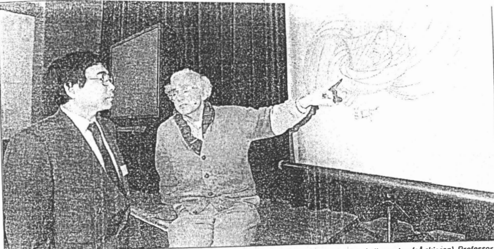
RADIOAKTIV? Fysiker David Fryberger tror Hessdalene-UFO'ene skyldes en radioaktiv partikkel han kaller vorton (på skissen). Professor Yoshi Ohtsuki mener elektromagnetisk interferens er årsaken.
