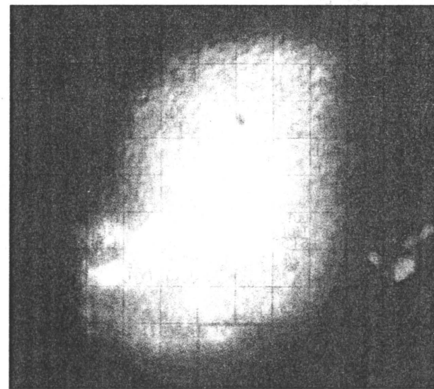
Et av UFO-fenomenene kraftig forstøttet. Kan dette være et plasmafenomen eller et kulelyn?
