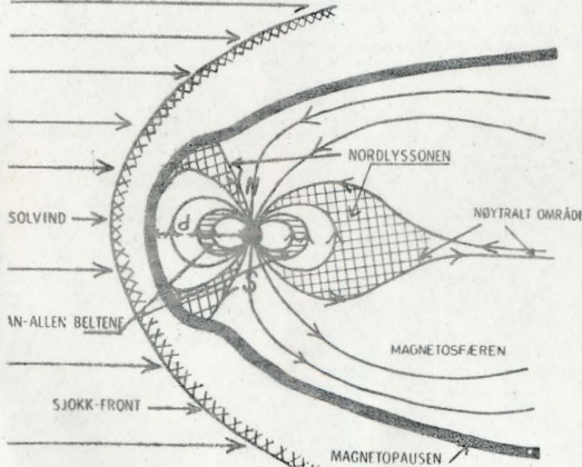
En modell av det nære verdensrom i et snitt gjennom solen og jorden. Den sorte kuleen midt i figuren representerer jorden.
