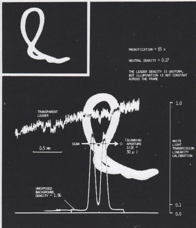
↓ Fig. 12. Mikrodensitometermåling af filmbilledet med det løkkeformede lys.
