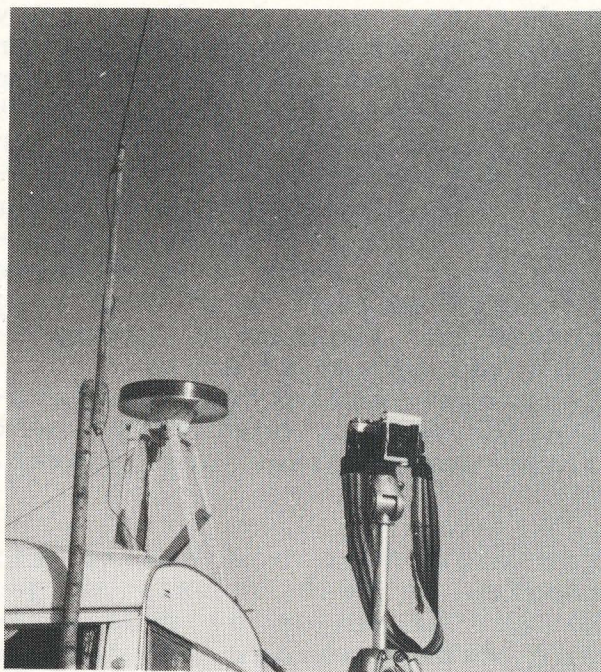
Kamera med gitter påmontert.
