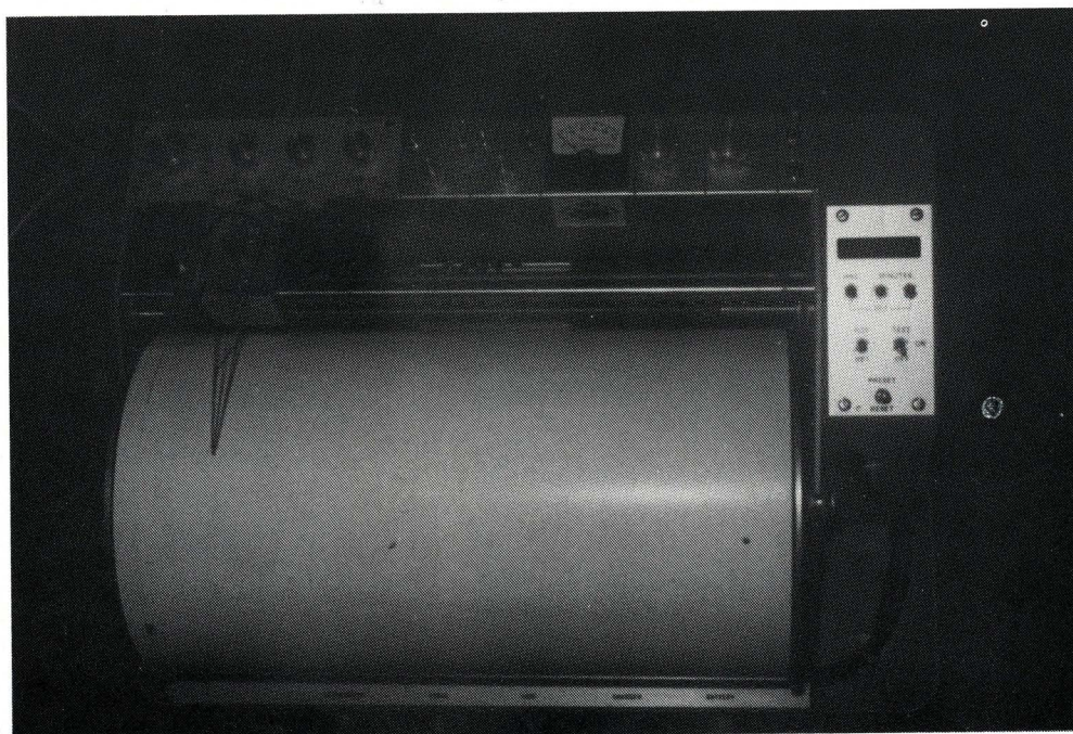
Seismografen, MEQ 800, som kan måle bevegelser i jordskorpa.
