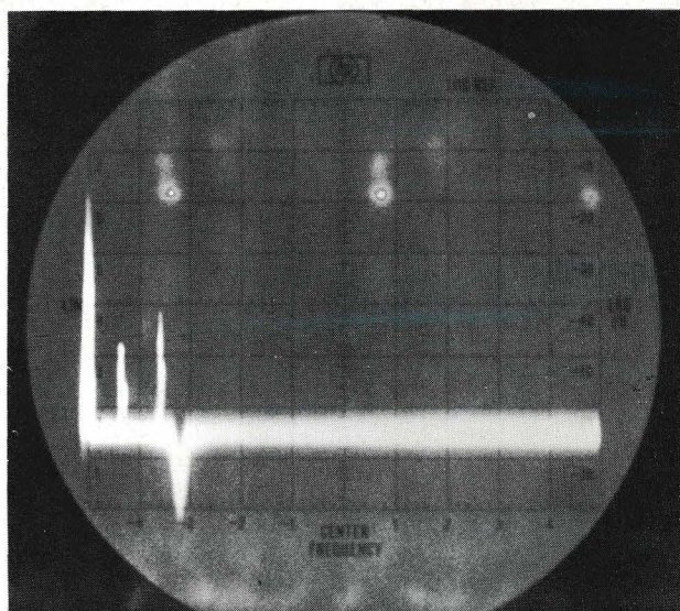
Skjermen på spektrumanalysatoren under "vanlige forhold" på dagtid. De 3 toppene til venstre viser AM-radiosignaler, FM-radiosignaler og TV-signalet.
