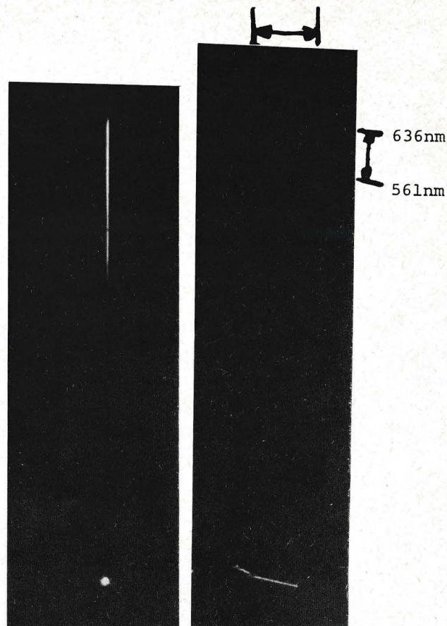
Sirius med 1.ordens spekter til venstre. Til høyre er det et ukjent lys.
