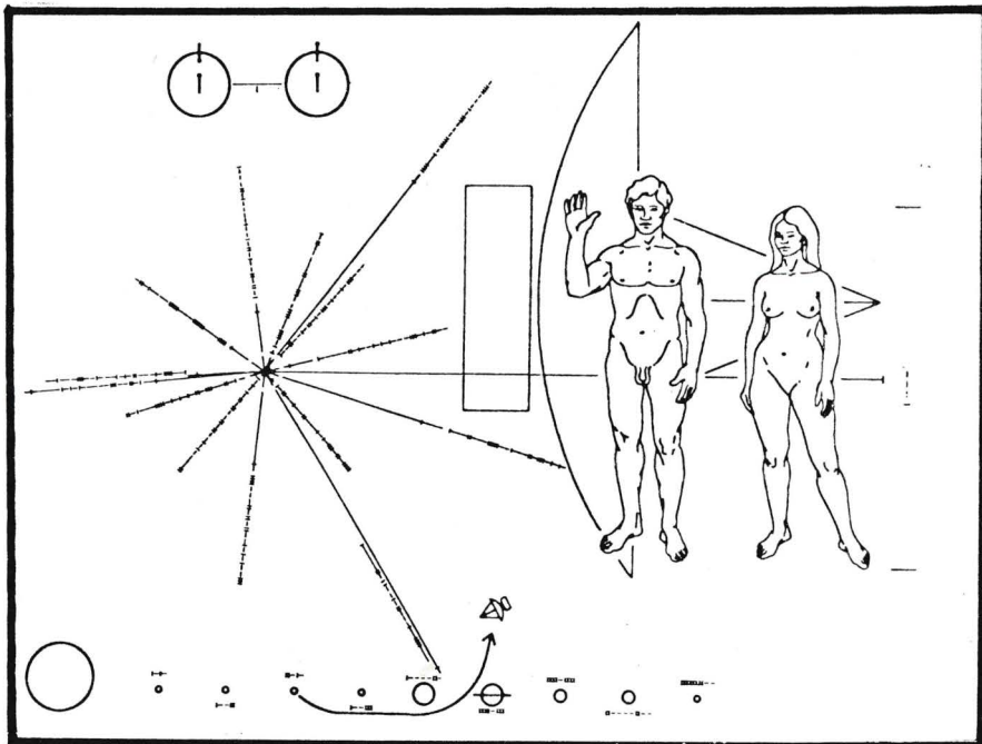
Kodemeldingen på Pioneer 10 antyder: Vannstoffatomets symbol øverst til venstre. Streksystemet viser til posisjoner på 14 pulsarer. Nederst vises sondens rute ut av solsystemet vårt, og slik ser altså mennesker ut idag.
