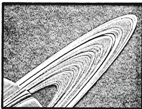
Dette bilde av Saturns ringer tok Voyager 1 fra en avstand av 8 millioner kilometer
