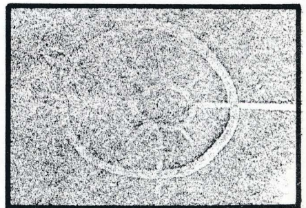
Dogontegning av planeten som kretser rundt Sirius C.
