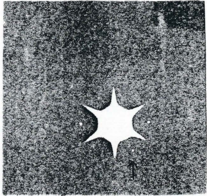
I året 1970 tok dr. Irving Lindenblad det aller første fotografi av Sirius B, som er den lille prikken nedenfor til høyre. De andre prikkene er reflekser fra linsene.
