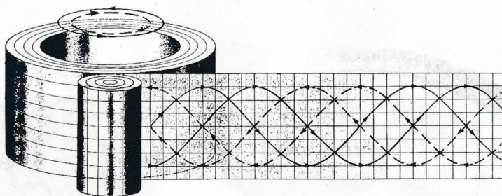
Fig. 7. Interaksjon mellom valse og ring: Båndet viser hvordan de virksomme krefter overlapper hverandre. Det er i alt 6 krefter, men av dem virker til enhver tid kun 4 sammen i hver omløpsretning: 2 likestrøms- og 2 vekselstrømskrefter. I valsene så vel som i ringene er de 2 forskjellige mulige vekselstrømmer faseforskjøvet 180 grader ( 1/2 fase) og kun aktive i den ene eller andre retning. Ved hver omløpsretning er den aktive vekselstrøm i valsen og den i ringen, som samvirker med den, faseforskjøvet 90 grader ( 1/4 fase). Ved motsatt omløpsretning tilsvarende med de to til enhver tid aktive, motsatt rettede vekselstrømmer.
