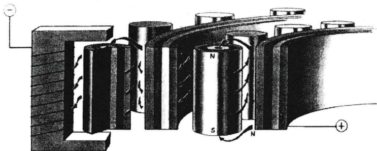
Fig. 1. Searl-effekt ved 4 \times 4 kvadrat. Bestanddelene i ringene såvel som i valsene er ordnet i lag: 1. elektronreservoar (lager), f.eks. neodym, 2. control gate (nylon 66), 3. akselerator, f.eks. Co, (Ag, Cu), 4. emitter, f.eks. Ti, (Mg). Ved 3 \times 3 kvadrat utelater man nylon-66 og ved 5 \times 5 kvadrat kommer ennå et akselerator-element i tillegg.
