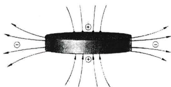
Fig. 4. Elektrostatisk potensial i radial retning, elektronstrømmen fra ringen til valse sett fra siden. Elektronavgivelsen fra valse og fra generatorene i sin helhet ligner et hjul, som sprøyter sentrifugalt, når gaten er våt av regn. Ringene beveger seg ikke, kun valse.
