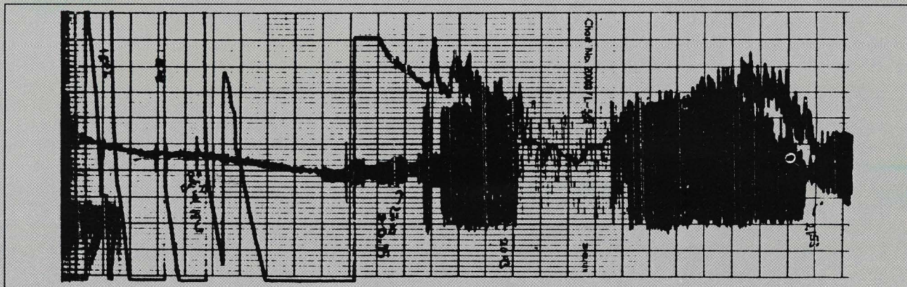
Grafen over viser en utskrift fra magnetometeret. De største utslagene måler 800 nanoTesla fra peak til peak, noe som er nesten 1000 ganger mer enn normalt.
