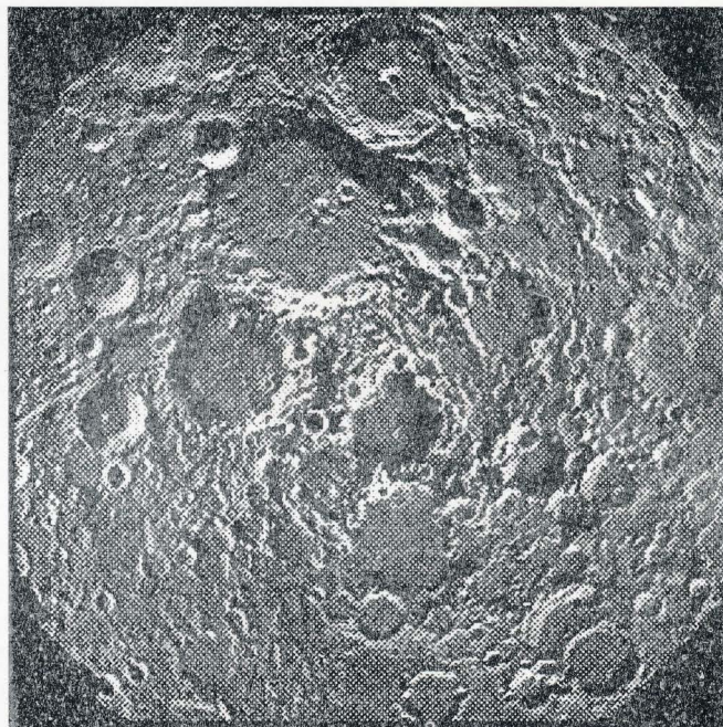
Foto av Månens sydpol, det såkalte Aitken-bassenget.
