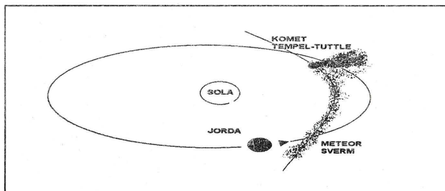
Illustrasjon som viser deler av komet Tempel-Tuttles bane rundt Solen.
