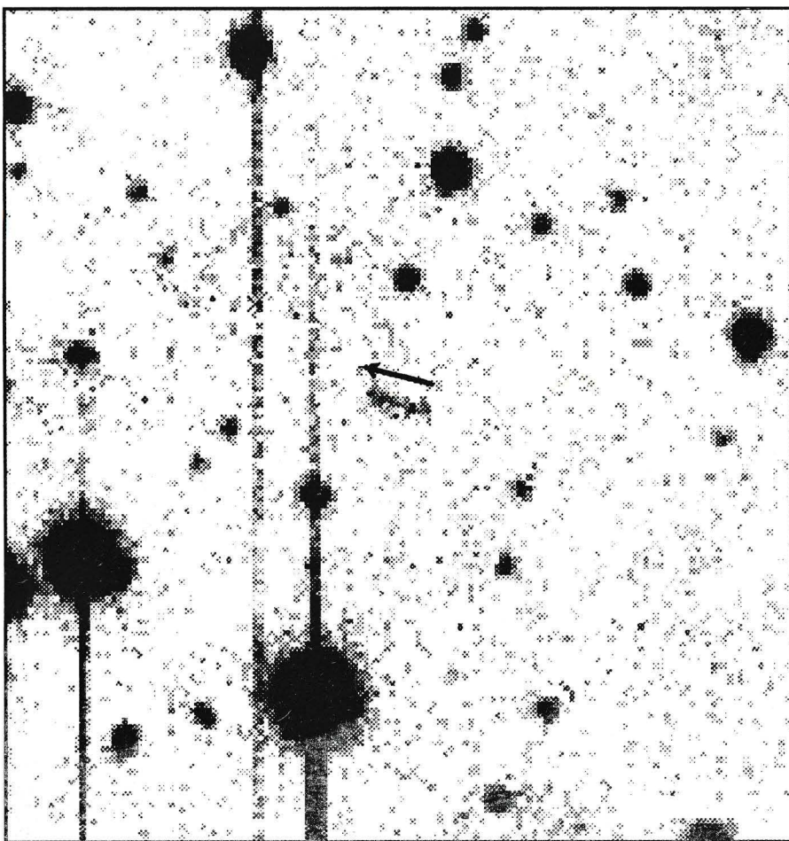
Asteroide 1997 XF 11 fotografert den 11. mars i år på tidseksponering. Den kan skimtes som en uklar strek under pilen midt på bildet. Fotoet (en CCD-negativ) er tatt den 11. mars gjennom 3,5 meter teleskopet ved Apache Point, New Mexico. Vertikale striper over og under nærliggende stjerner er artifakter fra optikken.
