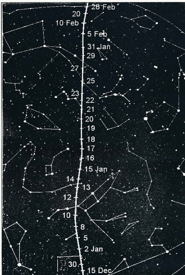
Til venstre: Tempel-Tuttles ferd over himmelen mellom 15. desember 1997 og 28. februar i år. Den 17. januar passerte den svært nær himmelens nordpol.
