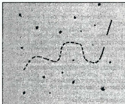
Figur 4. Objektets bane.
