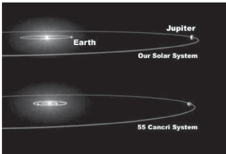
En sammenlikning av vår solsystem og 55 Cancri-systemet. (Foto: nasa.gov)
