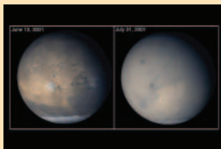
Utviklingen av en støvstorm på Mars
