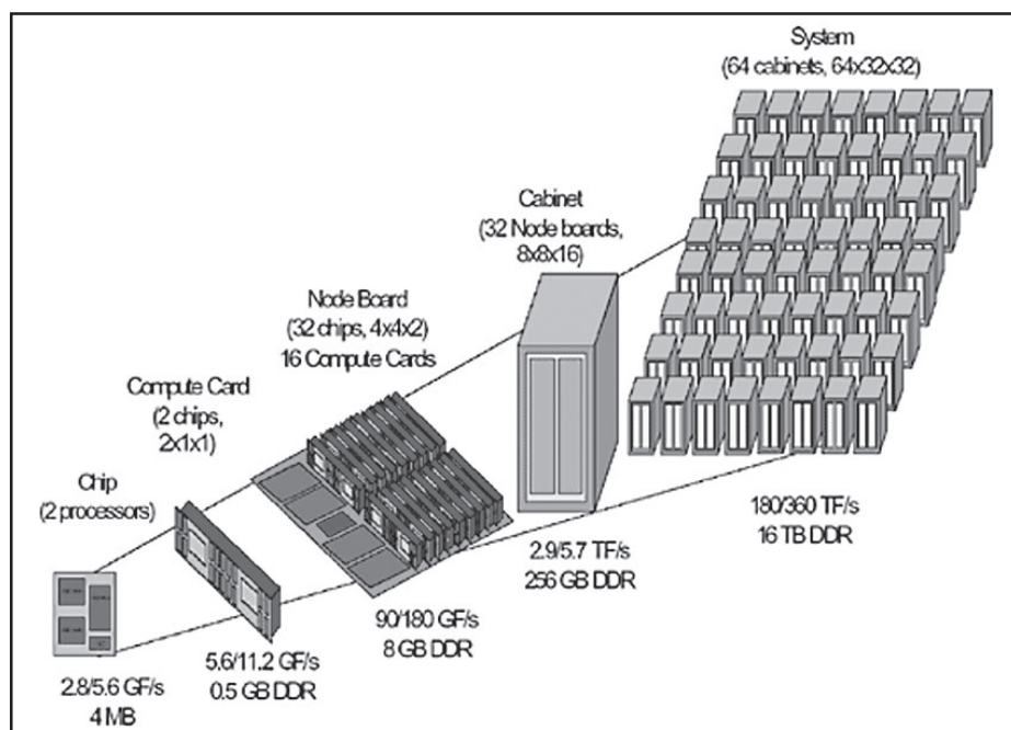
Prinsippskisse av Blue Gene.
