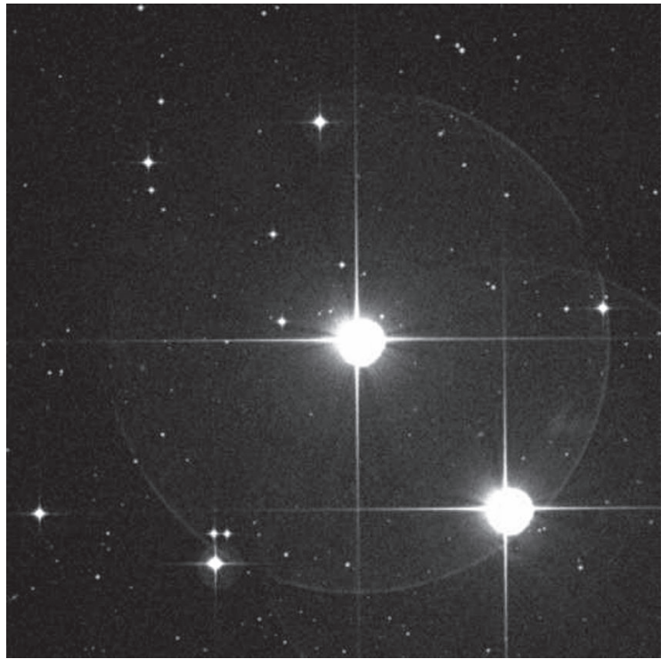
Zeta Reticuli 1 og 2
