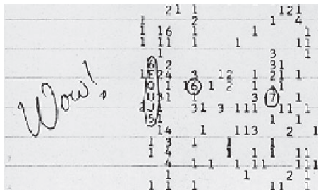
Det berømte «Wow!-signalet som ble registrert 15. august 1977.
