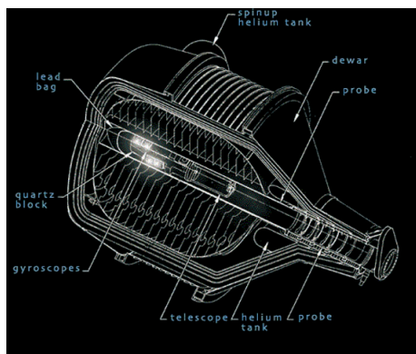
Oversiktstegning som viser Dewar-flasken med instrumentering.
