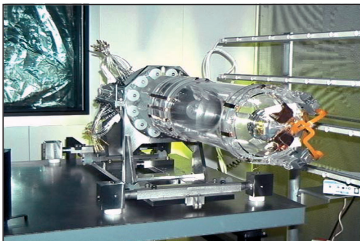
Teleskopet (foran) og gyroskopene (bak) bundet sammen i én kvartsblokk, kalt Science Instrument Assembly, SIA.
