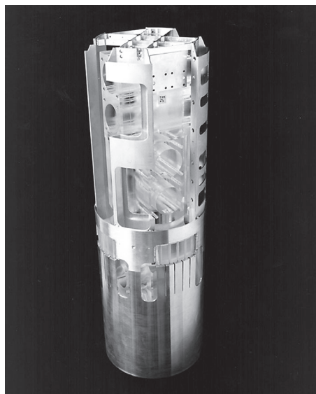
Kvartsblokken som huser de fire gyroskopene.
