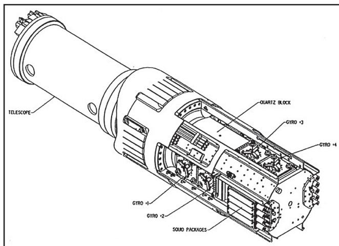
Teleskopet (foran) og gyroskopene (bak) bundet sammen i én kvartsblokk, kalt Science Instrument Assembly, SIA.
