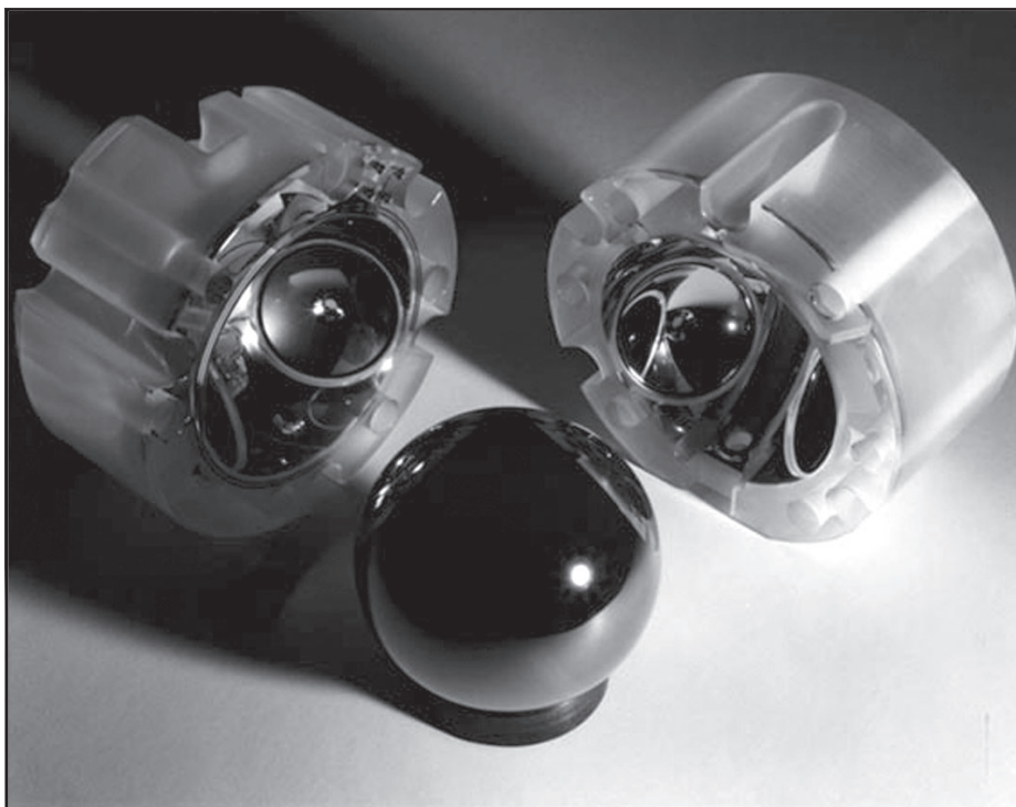
Kvartsblokken som huser de fire gyroskopene.
