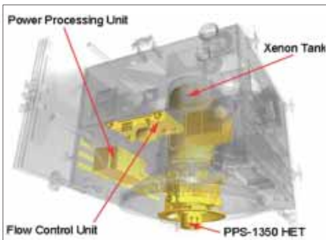
Skisse som viser ionemotoren (underst) sammen med xenon-tank og kontroll instrumenter
