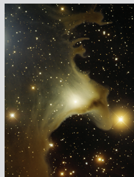
Forsidefoto/bakgrunn: Spøkelseståken i stjernebildet Cepheus. © T.A. Rector/University of Alaska Anchorage, H. Schweiker/WIYN and NOAO/AURA/NSF.
