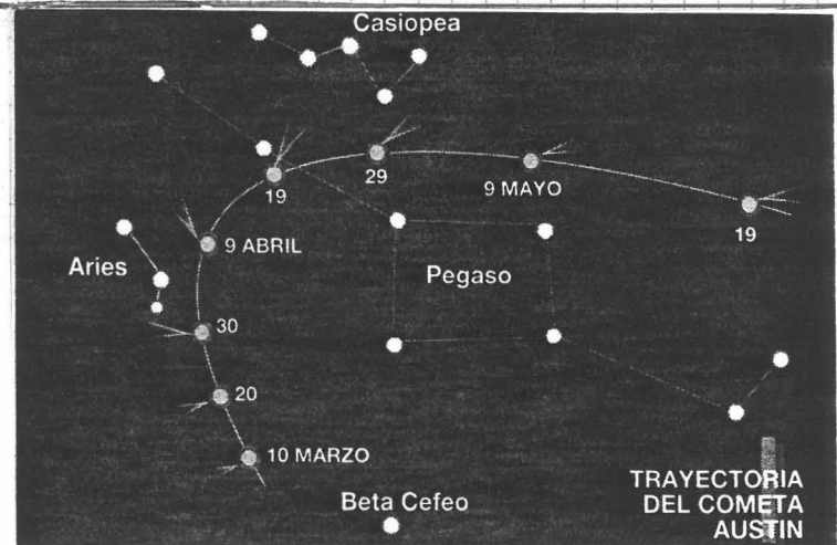
Trayectoria que seguirá el cometa Austin en su viaje solar.
