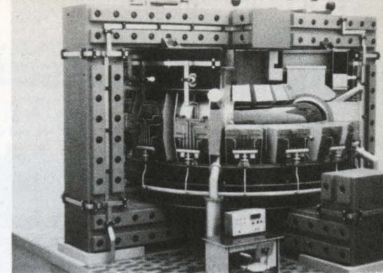
Den ryska fusionsreaktorn av Tokamak-typ.
