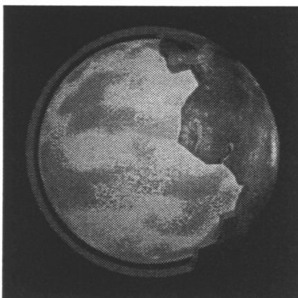
Mars – en del av skorpan har skalats bort och innandömet syns. Teckning: Thomas Feiner
