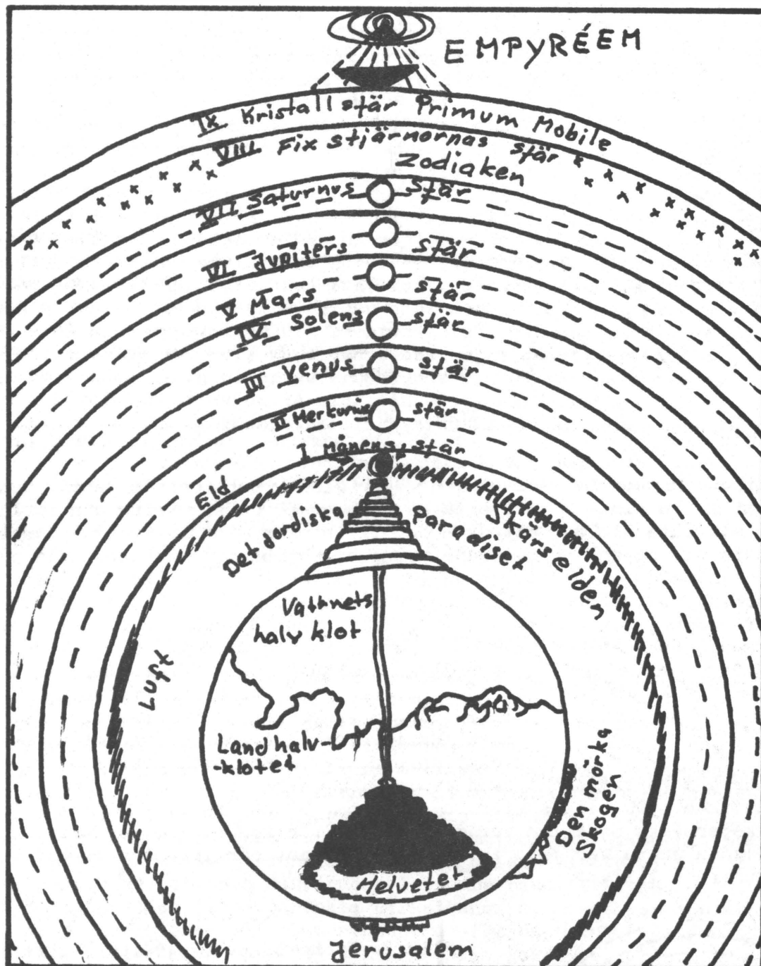
Bild 1. Aristoteles' (384-322 f Kr) världsbild, här som Dante uppfattade den, var uppbyggd i sfärer. Innerst fanns de fyra elementsfärerna, sedan kom 54 himmelssfärer och ytterst, omslutande världsalltet, rörde sig fixstjärnesfären.
