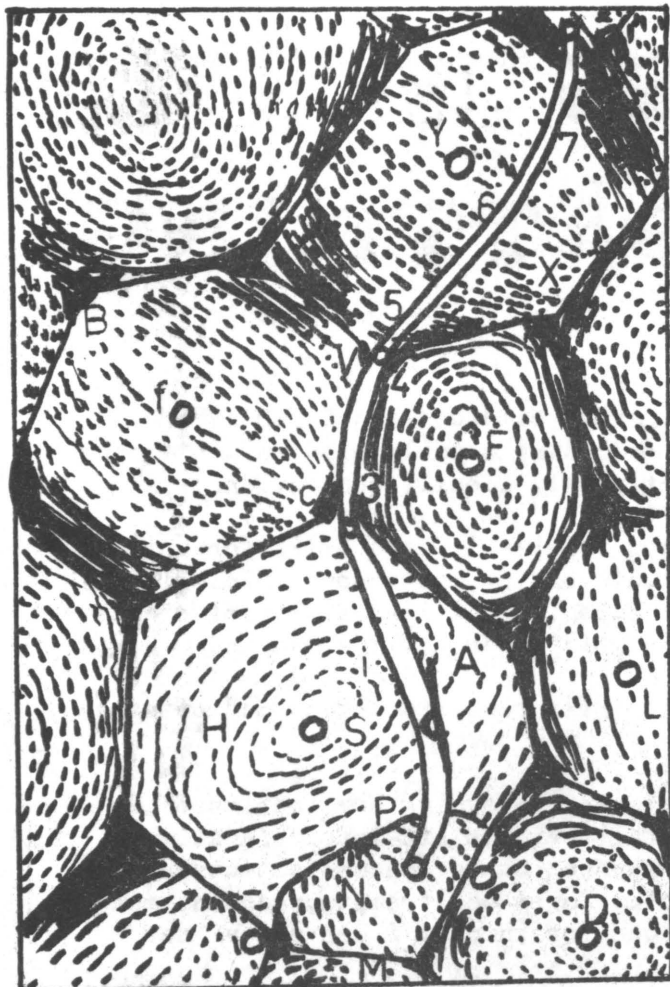
Bild 4: René Descartes (1596-1650) presenterade den sista stora sammanhängande kosmologin före Newton. Hans och Galileis studier av rörelsen kom att bilda en viktig grundval för Newton, medan hans teori om virvlarna och hans vägran att gå med på att det kan existera ett tommrum blev en av orsakerna till att Newton började arbetet med sin beskrivning av världsalltets byggnad.
