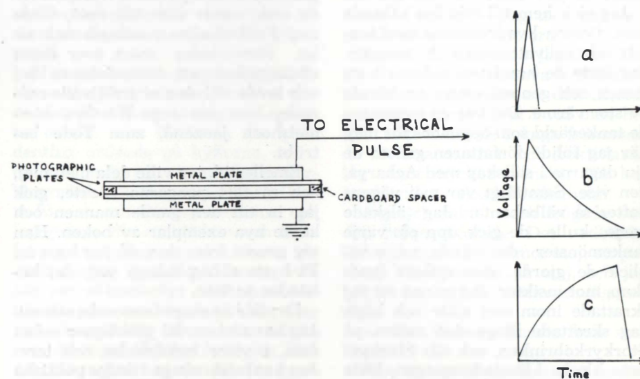
Bild 2. Den använda metoden att exponera den ljuskänsliga plåten för en elektrisk puls av någon av följande typer: (a) spikformad puls med snabb stegring och nedgång, (b) snabb stegring och långsam nedgång, (c) långsam stegring och snabb nedgång.
