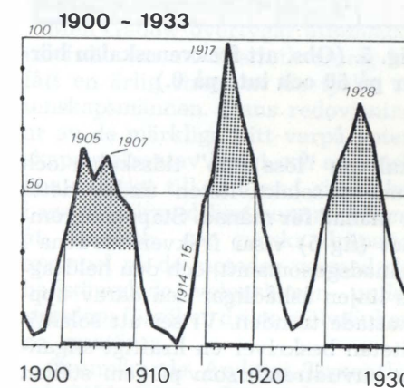
Fig. 3. Det skuggade området visar den del av solkurvan som är närmare max än min. Detta finns avsatt på tidsskalan nederst.
