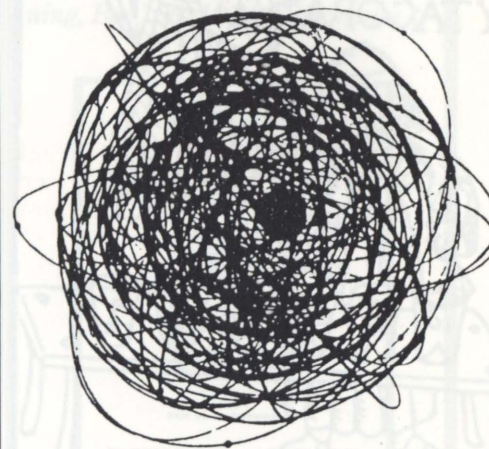
Elektronbanemodell för volframatom. Ur Folkvett.
