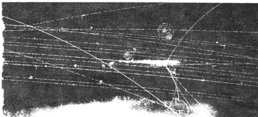
Pl. 5. Bubbelskärmbild av pion-myon-elektron-sönderfall. De två protonernas kollision resulterar i sex nya spår. De fyra nedre utgörs av pioner av vilka två sönderfaller. (Från Brookhaven National Laboratory, Upton, New York)
