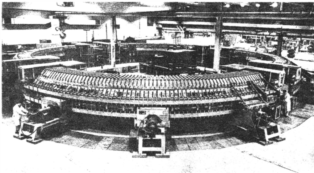
Pl. 3. Kosmotronen, en synkrotron som accelererar protoner i en cirkulär bana till hastigheter nära ljusets. (Från Brookhaven National Laboratory, Upton, New York)
