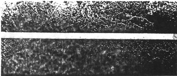
Radarbilden och ovan samma bild tolkad av data. Kanalerne syns tydligt.
