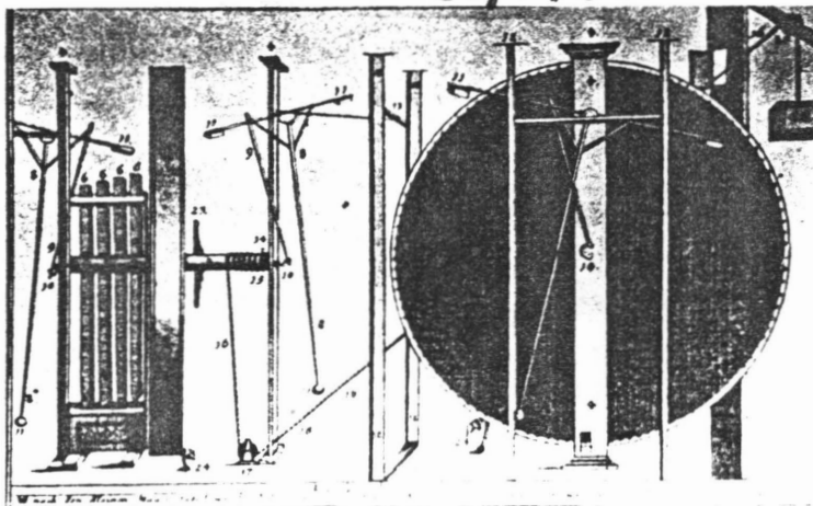
Detta är en ritning på Orffyreus evighetsmaskin ur en pamflett, som han själv gav ut 1715.
