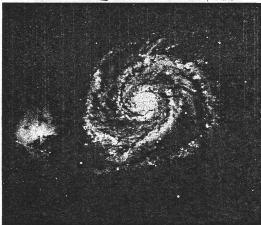
Det finns minst en miljard galaxer i rymden. Det här är en av dem, och kom ihåg att varje galax innehåller cirka 100 miljarder stjärnor.
