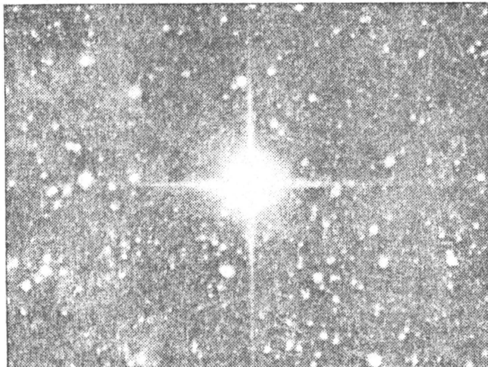
Supernova. År 1987 exploderade en stjärna i vår galax, den första sedan 1604.
