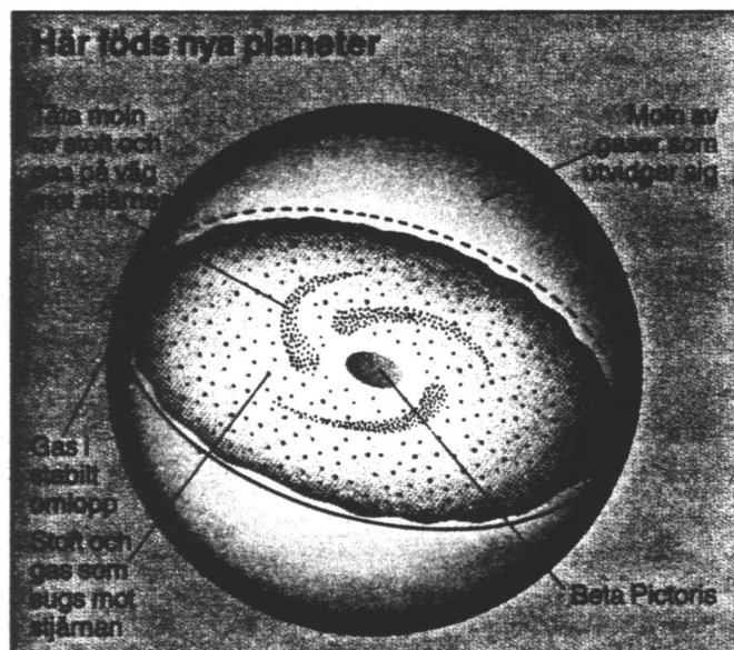
Molnen runt stjärnan Beta Pictoris tillförs hela tiden nytt stoft och nya gaser. Därför bildas det ett nytt planetsystem.
