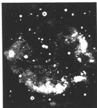
En supernova förlorar så mycket av tyngdkraften att dess planeter kan slitas loss.
