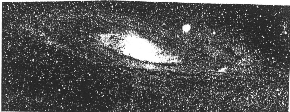
Först när astronomen Edwin Hubble omkring år 1920 mätte avståndet till vår granne Andromedagalaxen, fick man klart för sig att universum består av mer än en galax.
