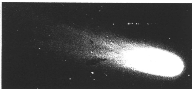
Kometsvansar bildas, när solvinden trycker bort gas och stoft från kometen. Därför blåser svansen bort från solen.
