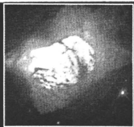
Solens sista tid kommer att bli som dödskampen hos stjärnan NGC 7027, 3 000 ljusår bort.
