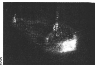
Gasskivan (grön) håller på att blåsas bort av ljus från stjärnan Theta 1 Orionis.
