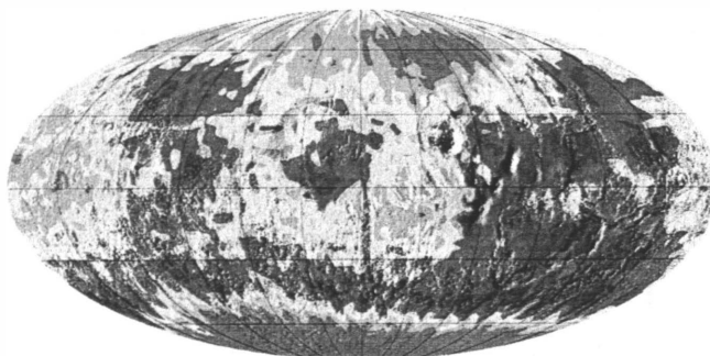
Marsvatten. De blå fläckarna visar var det finns väte på Mars. Vätet är med stor sannolikhet bundet i underjordiskt fruset vatten.
