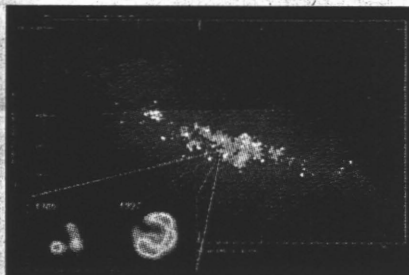
De här resterna av en supernova har fångats på bild tack vara VLBI-tekniken. Foto: EUROPEAN VLBI NETWORK
