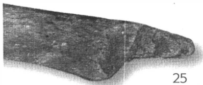
Isen smälter inte, för den ligger i skugga. Kraterns sidor är upp till två kilometer höga.
