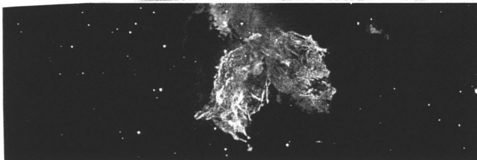
Supernovaresten N63A skapar en gigantisk gasexplosion, som skickar chockvågor genom rymden. Explosionen kan på sikt medföra att det föds nya stjärnor.
